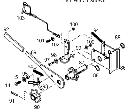
Left Winch Shown
