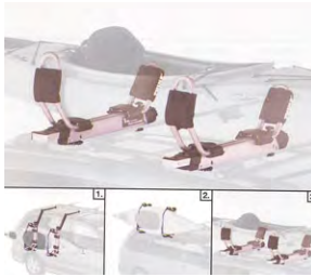
897XT - Hullavator
